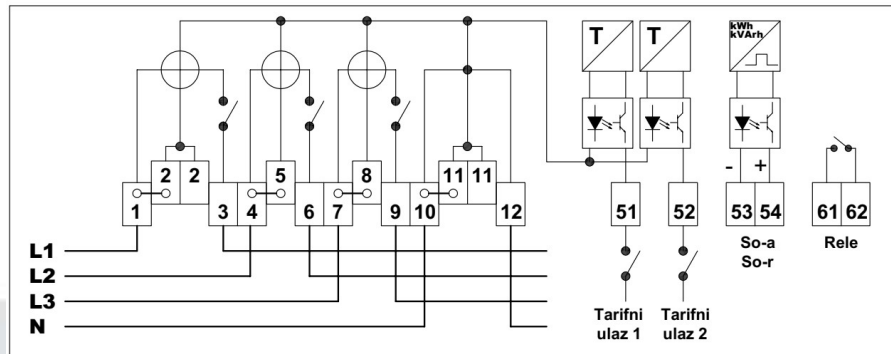
Slika 2.8 Šema povezivanja brojila tipa EWGE31x za direktan priključak sa internom sklopkom - varijanta 1
