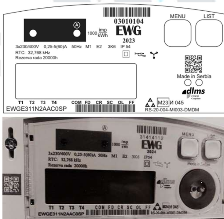
Slika 2.6 Natpisna ploča brojila tipa EWGE31x (gore na papiru, dole laserovano)
