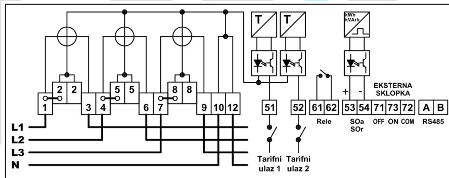
Slika 2.9 Šema povezivanja brojila tipa EWGE31x za direktan priključak varijanta 2
