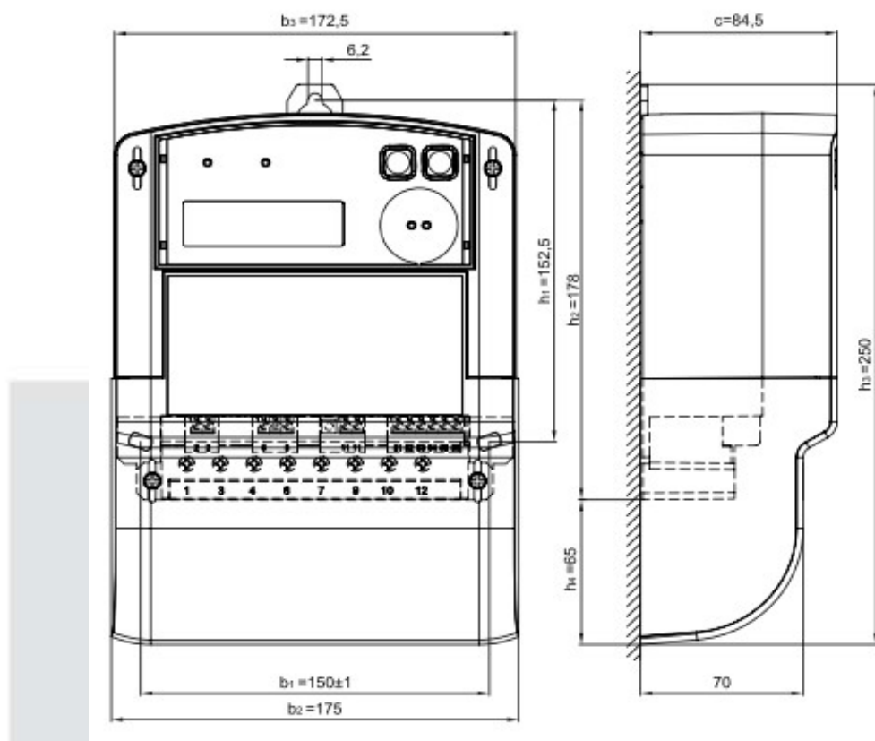
Slika 2.2. Dimenzije brojila
