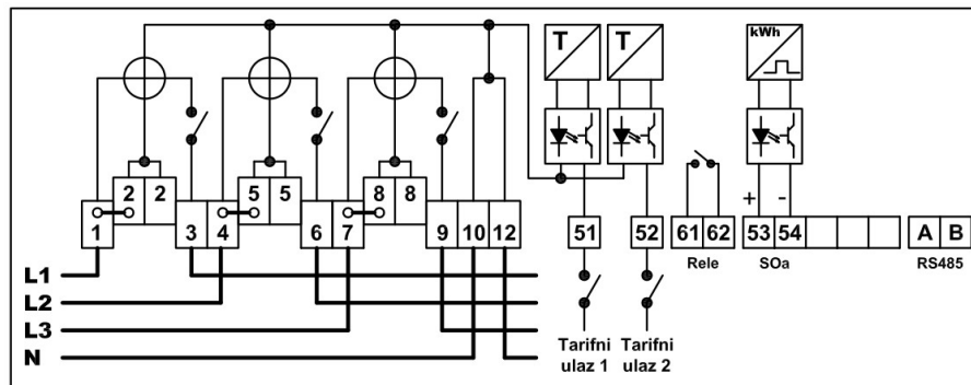
Slika 2.10 Šema povezivanja brojila tipa EWGE31x za direktan priključak sa internom sklopkom - varijanta 2
